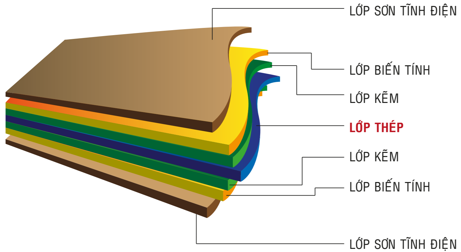
CHI TIẾT CẤU TẠO CỬA KÉO
